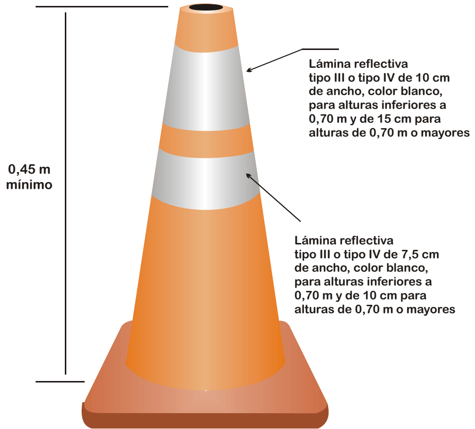
Figura 4.2 Conos
