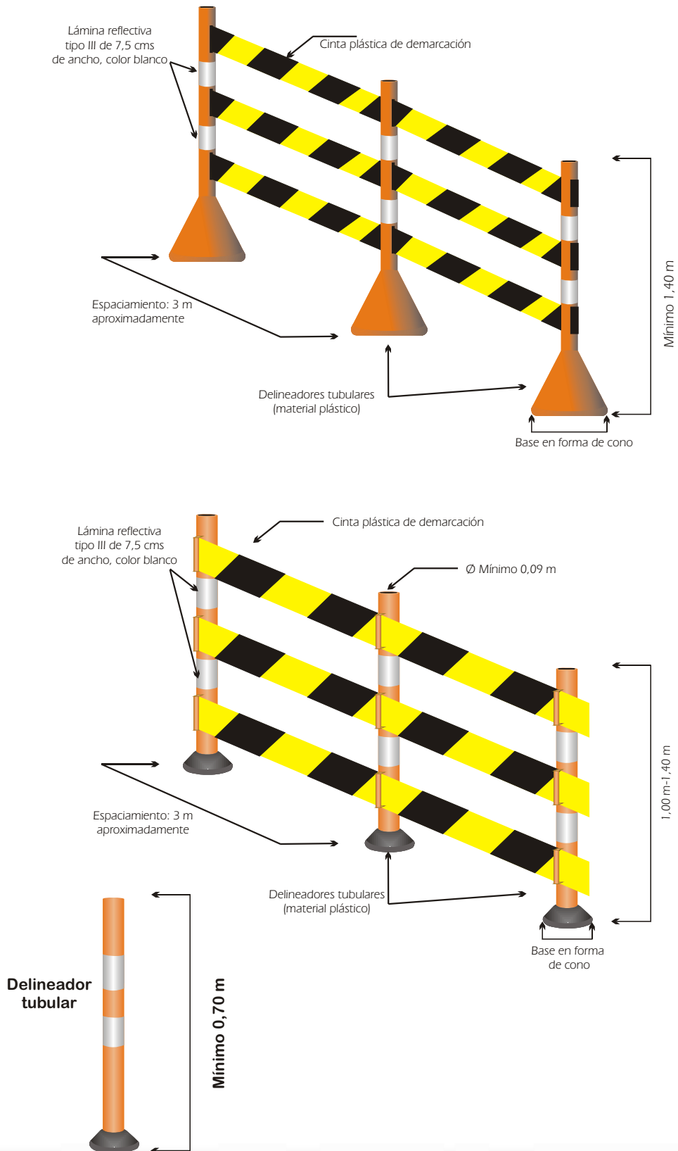
Figura 4.3 Delineadores tubulares
